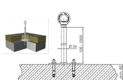
Betonilaatan ankkurointipiste (ASP EV2)
