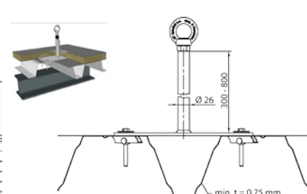
Kantavan poimulevyn ankkurointipiste (ASP EV9)
