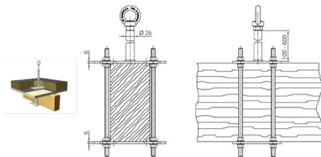
Liimapuupalkin ankkurointipiste (ASP EV5)
