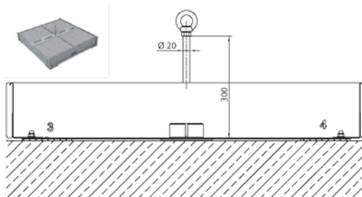
LUX-top® mobile -ankkurointipiste
