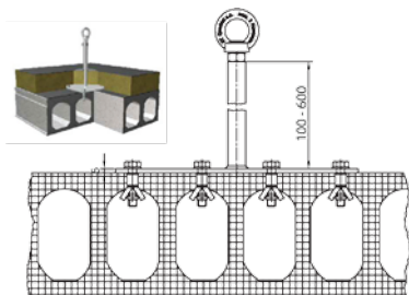
Ontelolaatan ankkurointipiste (ASP EV10)
